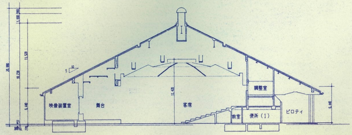
断面図(YH6通り)
